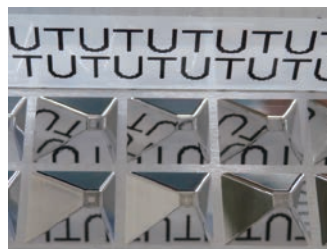
Surface roughness 15° Ra 0.014 μm 45° Ra 0.018 μm
