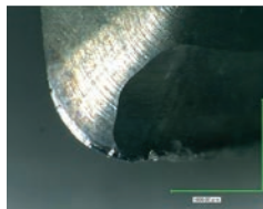
Rake Face
